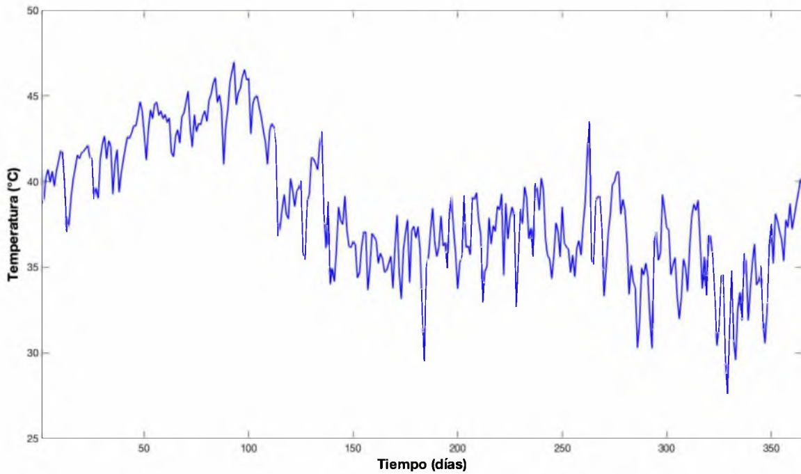
Figura 58. Perfil diario de temperatura promedio en la salida de los colectores solares de placa plana para una simulación de un año (365 días) contemplando el escenario uno ( 36 \text{ m}^2 ).
