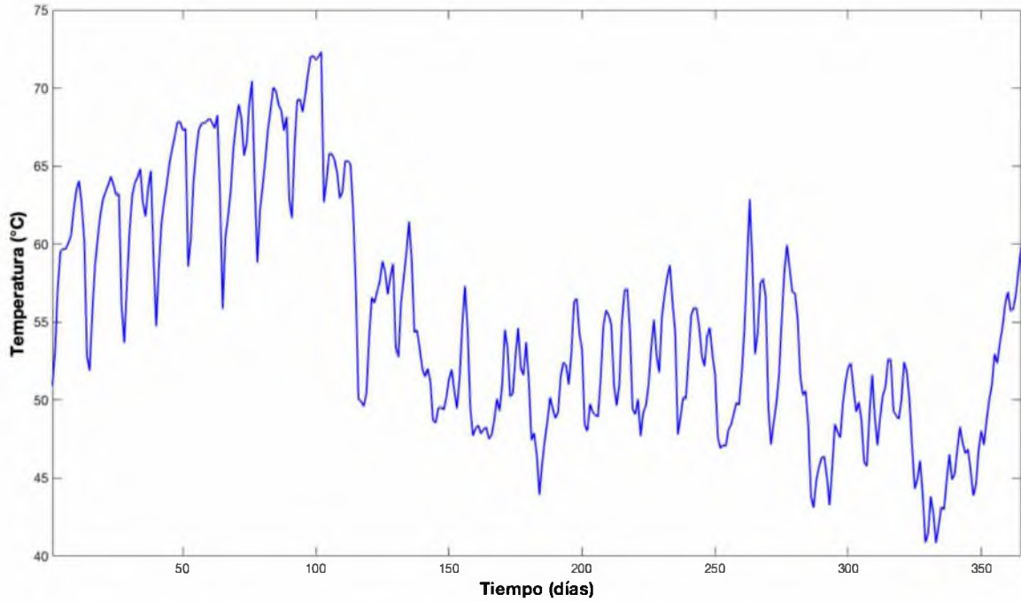
Figura 63. Perfil diario de temperatura promedio en el tanque de almacenamiento de energía térmica para una simulación de un año (365 días) contemplando el escenario dos ( 24 \text{ m}^2 ).
