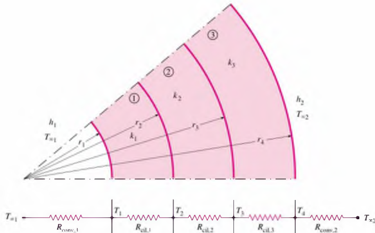
Figura 22. Red de resistencias térmicas para la transferencia de calor a través de un cilindro compuesto de tres capas sujeto a convección en ambos lados [15].
