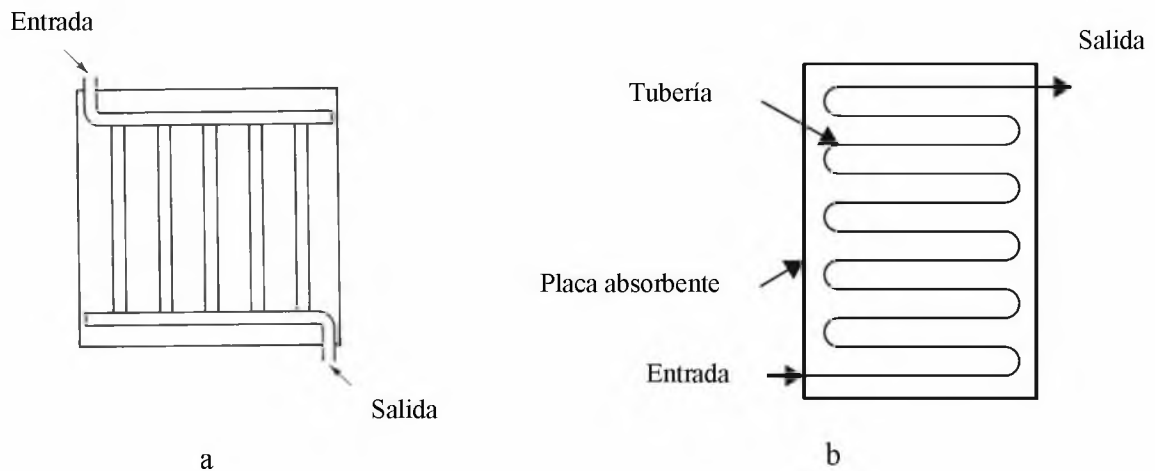
Figura 16. Configuraciones de la tubería de transporte del fluido de trabajo. a) Tubos paralelos con distribuidor. Modificado de [22]. b) Forma de serpiente. Modificado de [27].
