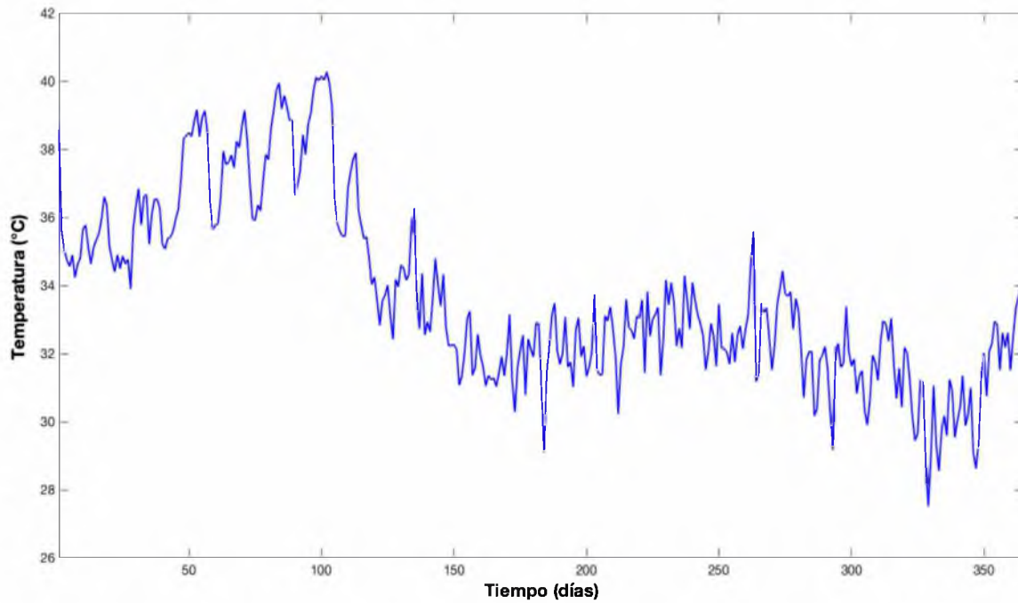
Figura 64. Perfil diario de temperatura promedio en la salida de los colectores solares de placa plana para una simulación de un año (365 días) contemplando el escenario tres (12 m 2 ).
