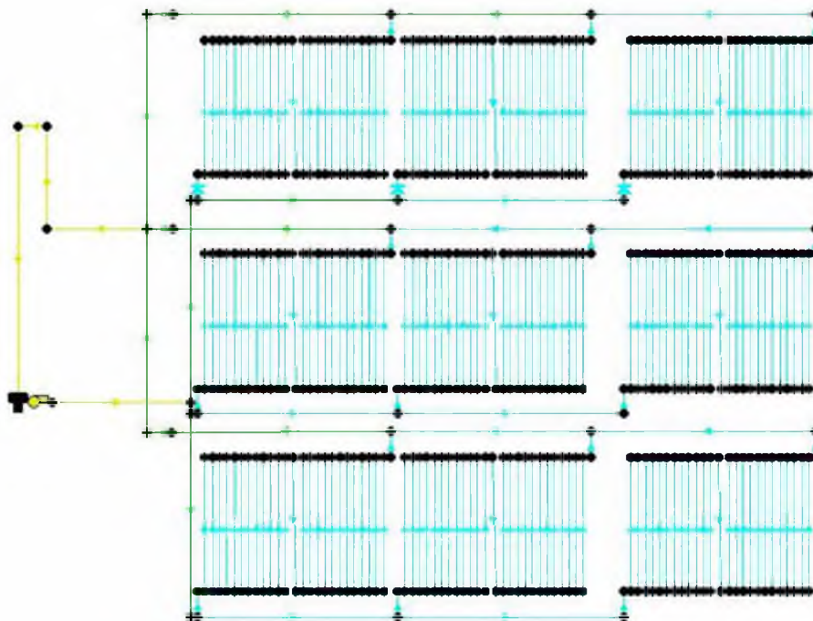
Figura 46. Esquema de la simulación hidráulica efectuada en el programa EPANET para determinación de flujos volumétricos en cada uno de los módulos del sistema de conducción de fluido de trabajo en los colectores solares.
