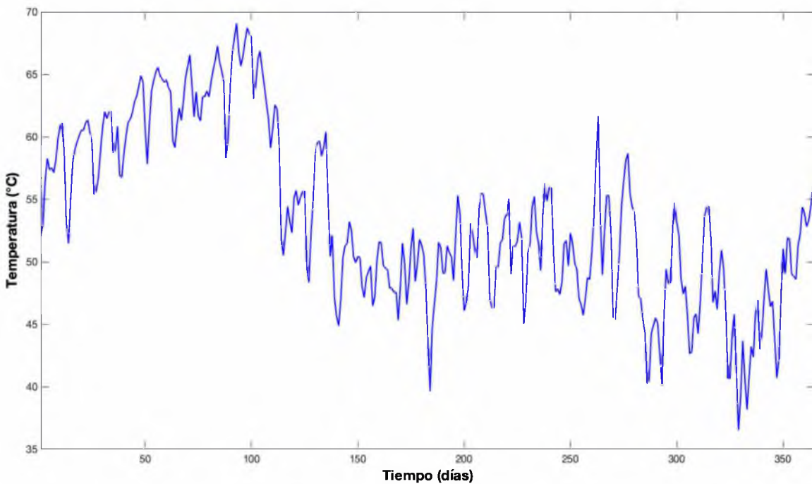
Figura 59. Perfil diario de temperatura promedio en el tanque de almacenamiento presurizado para una simulación de un año (365 días) contemplando el escenario uno ( 36 \text{ m}^2 ).
