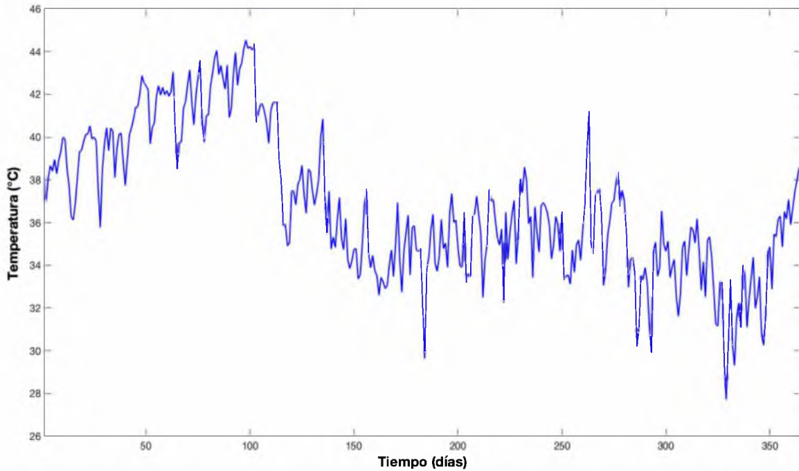
Figura 61. Perfil diario de temperatura promedio en la salida de los colectores solares de placa plana para una simulación de un año (365 días) contemplando el escenario dos (24 m 2 ).
