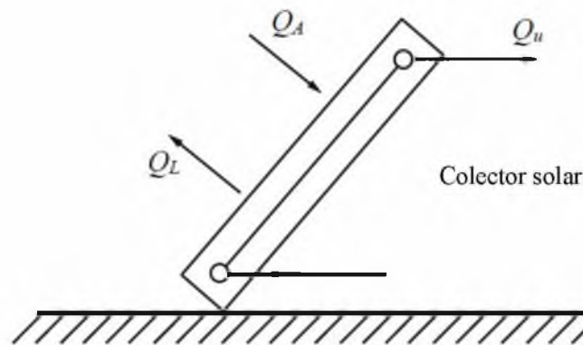
Figura 21. Esquema del balance energético en un colector solar de placa plana, donde Q_A corresponde a la energía que incide sobre la placa del colector solar, Q_u es la energía neta aprovechable y Q_L es la energía que se pierde a los alrededores. Modificado de [23].
